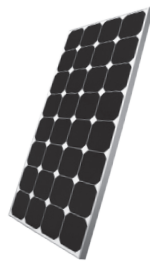
4x275w (1.1kW total) Mono Crystalline Solar Panels
